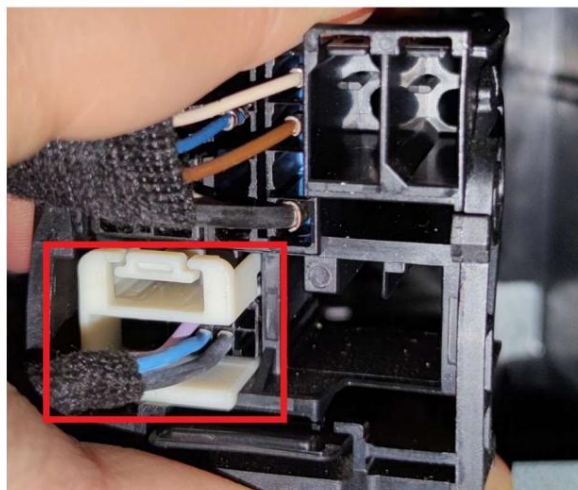
Złącza od strony konsoli środkowej
